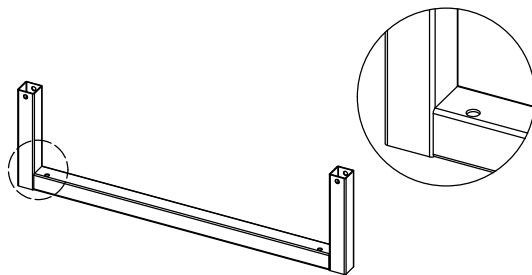
Poutre inférieure - Avant
