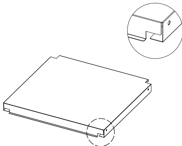
Panneau du bas
