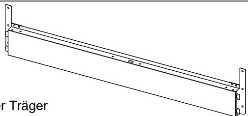
Oberer Träger
